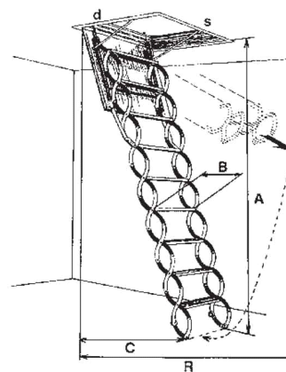
Principtegning af Lusso PP
