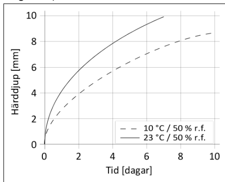
Diagram 1: Härdningshastighet Sikaflex®-295 UV
