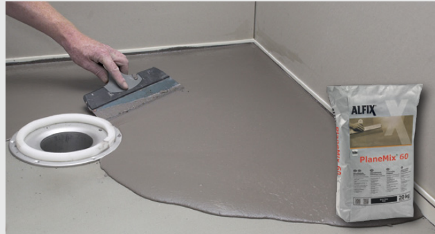
Fallupbyggnad vid traditionellt golvbrunn
