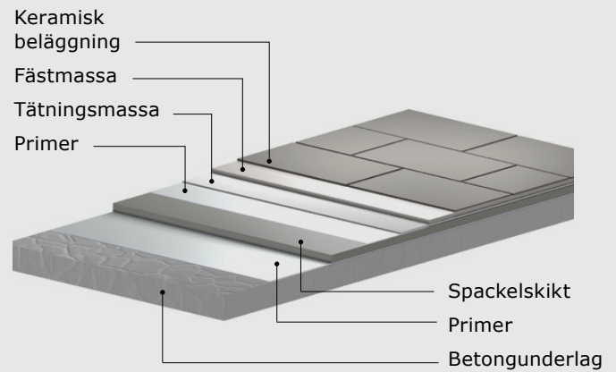
Utomhus spackling på betongunderlag
