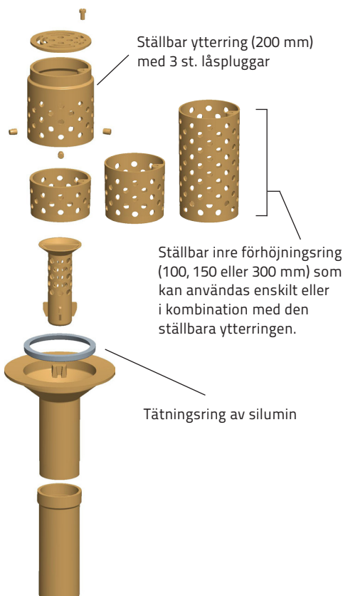
Bild 1 TG-brunn 4" med ställbar förhöjningsring samt plansil.
